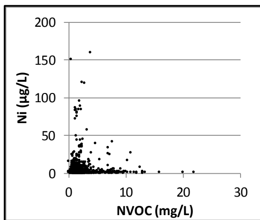
Bilag 17. Lokalenhed Sjælland. Nikkel (Ni) vs dybde, nikkel og pH, nikkel og ilt (O 2 ), nikkel og nitrat (NO 3 ) samt nikkel og NVOC. Data er indsamlet i perioden 1993-2013 fra aktive borer i 2013. Koncentrationer under detektionsgrænsen er vist med den numeriske værdi.
