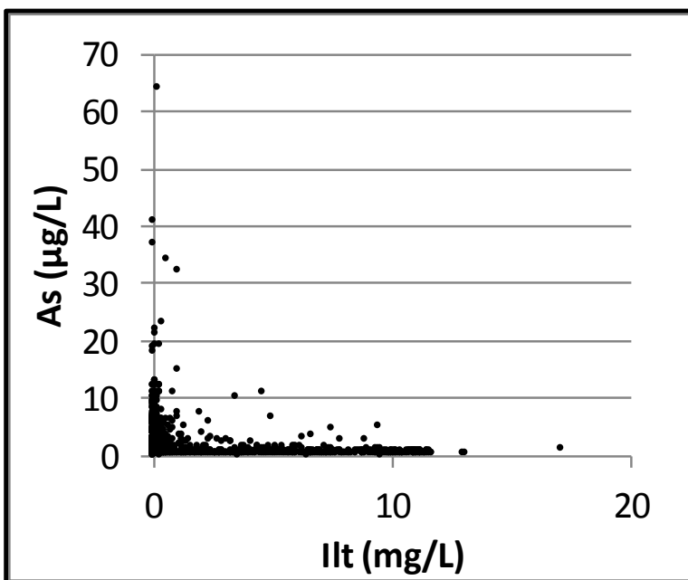
Bilag 8. Lokalenhed Sjælland. Arsen vs dybde samt arsen og ilt ( \text{O}_2 ). Data er indsamlet i perioden 1993-2013 fra aktive boringer i 2013. Koncentrationer under detektionsgrænsen er vist med den numeriske værdi.
