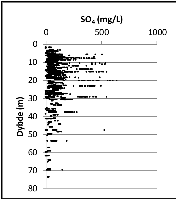
Bilag 6. Lokalenhed Sjælland. Sulfat ( \text{SO}_4 ) vs. dybde. Data er indsamlet i perioden 1993-2013 fra aktive boringer i 2013. Koncentrationer under detektionsgrænsen er vist med den numeriske værdi.
