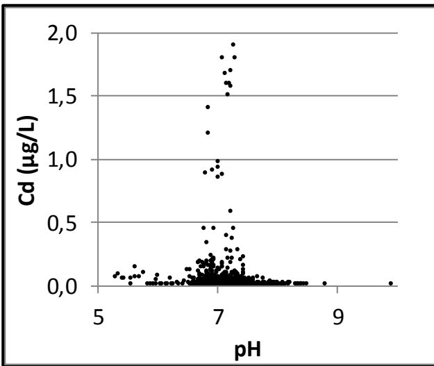
Bilag 13. Lokalenhed Sjælland. Cadmium (Cd) vs dybde, cadmium og pH samt cadmium og NVOC. Data er indsamlet i perioden 1993-2013 fra aktive boringer i 2013. Koncentrationer under detektionsgrænsen er vist med den numeriske værdi.
