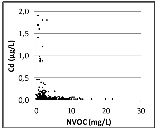
Bilag 13. Lokalenhed Sjælland. Cadmium (Cd) vs dybde, cadmium og pH samt cadmium og NVOC. Data er indsamlet i perioden 1993-2013 fra aktive boringer i 2013. Koncentrationer under detektionsgrænsen er vist med den numeriske værdi.
