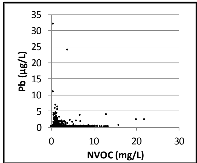
Bilag 18. Lokalenhed Sjælland. Bly (Pb) vs dybde, bly og pH samt bly og NVOC. Data er indsamlet i perioden 1993-2013 fra aktive boringer i 2013. Koncentrationer under detektionsgrænsen er vist med den numeriske værdi.
