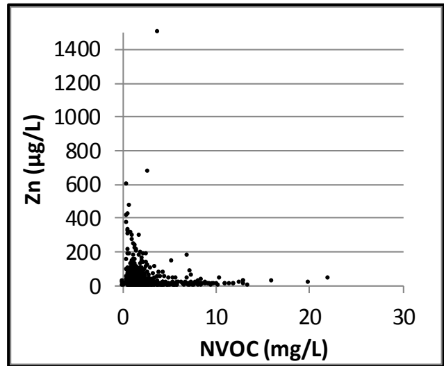
Bilag 19. Lokalenhed Sjælland. Zink (Zn) vs dybde, zink og pH samt zink og NVOC. Data er indsamlet i perioden 1993-2013 fra aktive boringer i 2013. Koncentrationer under detektionsgrænsen er vist med den numeriske værdi.
