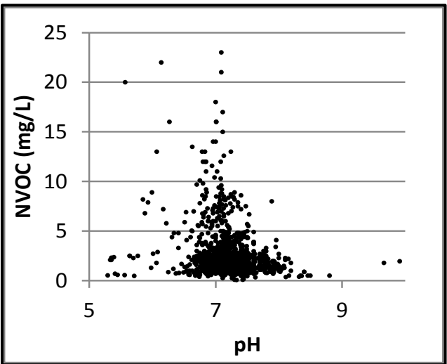
Bilag 4. Lokalenhed Sjælland. NVOC vs. dybde, NVOC og ilt (O 2 ) samt NVOC og pH. Data er indsamlet i perioden 1993-2013 fra aktive boringer i 2013. Koncentrationer under detektionsgrænsen er vist med den numeriske værdi.
