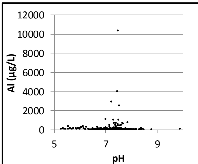
Bilag 7. Lokalenhed Sjælland. Aluminium (Al) vs dybde samt aluminium og pH. Data er indsamlet i perioden 1993-2013 fra aktive borer i 2013. Koncentrationer under detektionsgrænsen er vist med den numeriske værdi.
