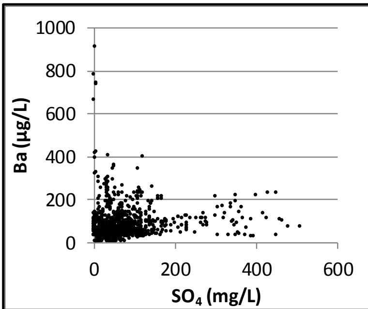
Bilag 10. Lokalenhed Sjælland. Barium vs dybde samt barium og sulfat (SO 4 ). Data er indsamlet i perioden 1993-2013 fra aktive boringer i 2013. Koncentrationer under detektionsgrænsen er vist med den numeriske værdi.
