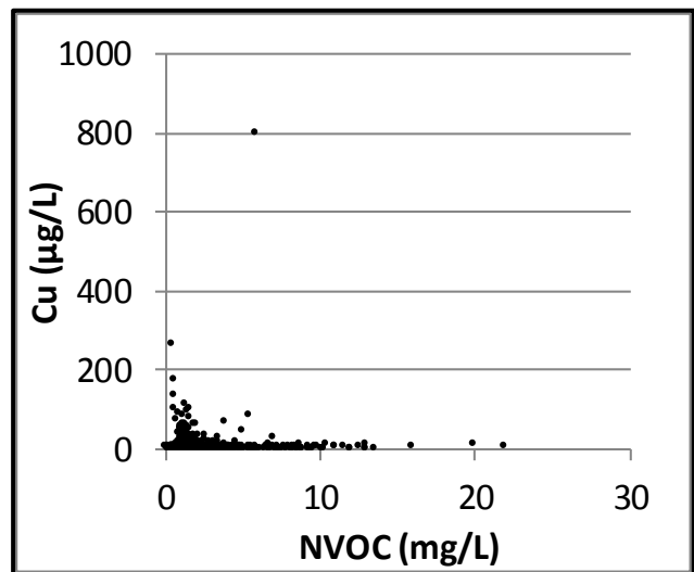
Bilag 14. Lokalenhed Sjælland. Kobber (Cu) vs dybde, kobber og pH samt kobber og NVOC. Data er indsamlet i perioden 1993-2013 fra aktive boringer i 2013. Koncentrationer under detektionsgrænsen er vist med den numeriske værdi.
