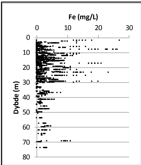
Bilag 2. Lokalenhed Sjælland. Redox potentiale, ilt og jern vs dybde. Data er indsamlet i perioden 1993-2013 fra aktive boringer i 2013. Koncentrationer under detektionsgrænsen er vist med den numeriske værdi.
