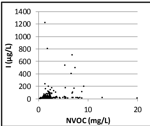
Bilag 16. Lokalenhed Sjælland. Jod (I) vs dybde, jod og NVOC samt jod og chlorid (Cl). Data er indsamlet i perioden 1993-2013 fra aktive boringer i 2013. Koncentrationer under detektionsgrænsen er vist med den numeriske værdi.
