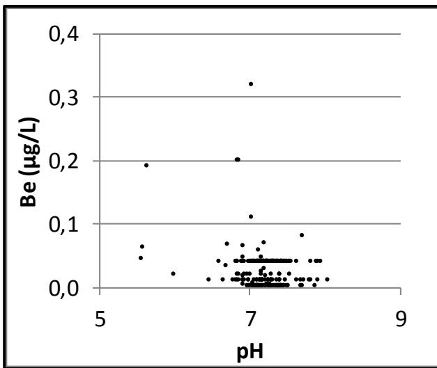
Bilag 11. Lokalenhed Sjælland. Beryllium (Be) vs dybde, beryllium og pH samt beryllium og NVOC. Data er indsamlet i perioden 1993-2013 fra aktive boringer i 2013. Koncentrationer under detektionsgrænsen er vist med den numeriske værdi.
