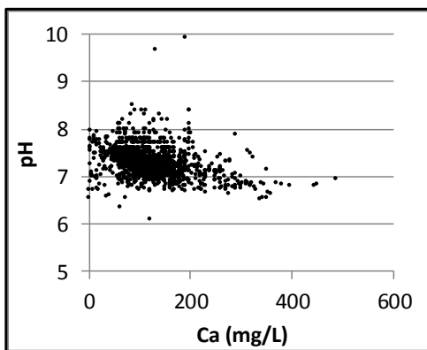
Bilag 1. Lokalenhed Sjælland. pH, hydrogencarbonat ( \text{HCO}_3 ) og calcium (Ca) vs dybde, pH og hydrogencarbonat samt pH og calcium. Data er indsamlet i perioden 1993-2013 fra aktive borer i 2013. Koncentrationer under detektionsgrænsen er vist med den numeriske værdi.
