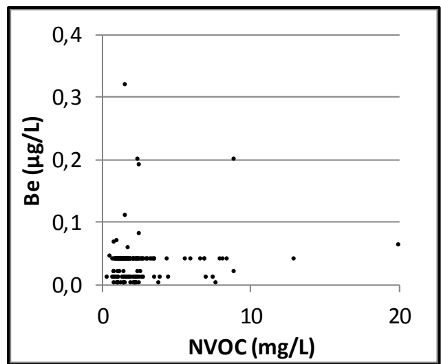
Bilag 11. Lokalenhed Sjælland. Beryllium (Be) vs dybde, beryllium og pH samt beryllium og NVOC. Data er indsamlet i perioden 1993-2013 fra aktive boringer i 2013. Koncentrationer under detektionsgrænsen er vist med den numeriske værdi.
