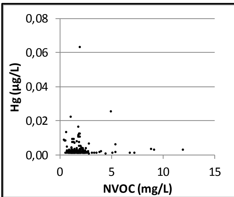
Bilag 15. Lokalenhed Sjælland. Kviksølv (Hg) vs dybde og kviksølv og NVOC. Data er indsamlet i perioden 1993-2013 fra aktive borer i 2013. Koncentrationer under detektionsgrænsen er vist med den numeriske værdi.
