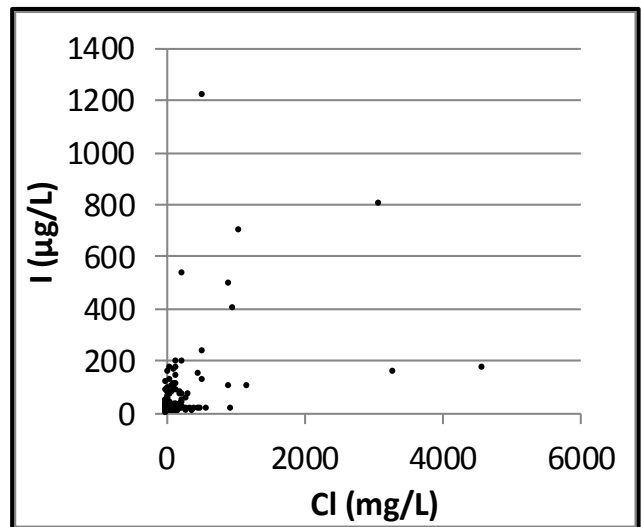
Bilag 16. Lokalenhed Sjælland. Jod (I) vs dybde, jod og NVOC samt jod og chlorid (Cl). Data er indsamlet i perioden 1993-2013 fra aktive boringer i 2013. Koncentrationer under detektionsgrænsen er vist med den numeriske værdi.
