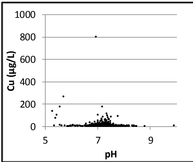
Bilag 14. Lokalenhed Sjælland. Kobber (Cu) vs dybde, kobber og pH samt kobber og NVOC. Data er indsamlet i perioden 1993-2013 fra aktive boringer i 2013. Koncentrationer under detektionsgrænsen er vist med den numeriske værdi.
