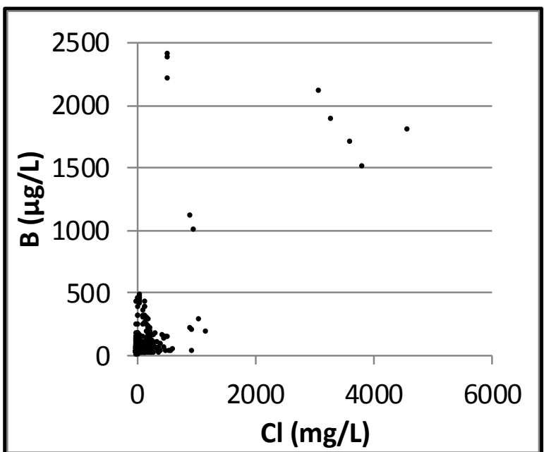
Bilag 9. Lokalenhed Sjælland. Bor (B) vs dybde samt bor og chlorid (Cl). Data er indsamlet i perioden 1993-2013 fra aktive boringer i 2013. Koncentrationer under detektionsgrænsen er vist med den numeriske værdi.
