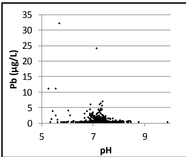
Bilag 18. Lokalenhed Sjælland. Bly (Pb) vs dybde, bly og pH samt bly og NVOC. Data er indsamlet i perioden 1993-2013 fra aktive boringer i 2013. Koncentrationer under detektionsgrænsen er vist med den numeriske værdi.
