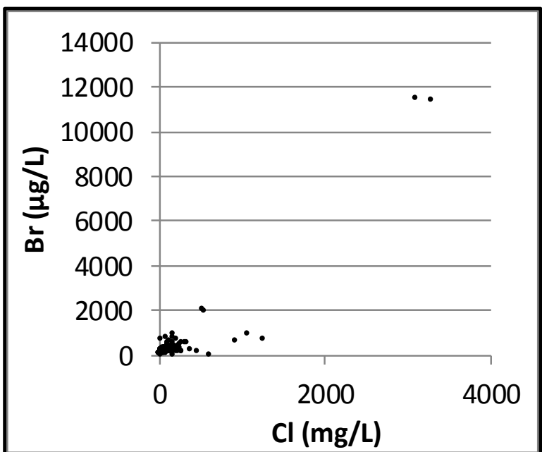
Bilag 12. Lokalenhed Sjælland. Brom (Br) vs dybde samt brom og chlorid (Cl). Data er indsamlet i perioden 1993-2013 fra aktive borer i 2013. Koncentrationer under detektionsgrænsen er vist med den numeriske værdi.
