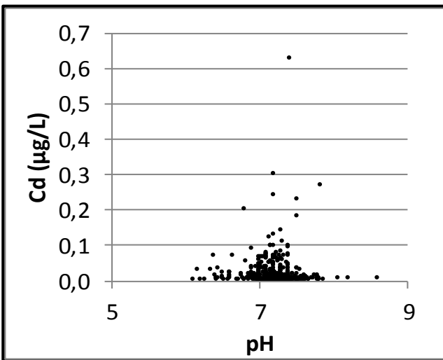
Bilag 13. Lokalenhed Fyn. Cadmium (Cd) vs dybde, cadmium og pH samt cadmium og NVOC. Data er indsamlet i perioden 1993-2013 fra aktive boringer i 2013. Koncentrationer under detektionsgrænsen er vist med den numeriske værdi.
