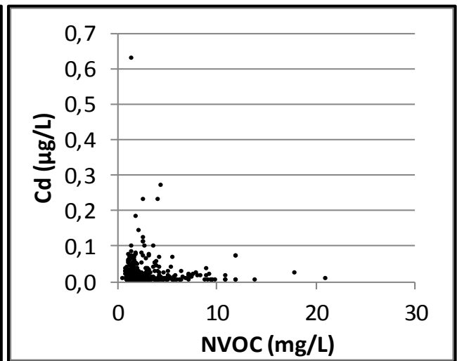
Bilag 13. Lokalenhed Fyn. Cadmium (Cd) vs dybde, cadmium og pH samt cadmium og NVOC. Data er indsamlet i perioden 1993-2013 fra aktive boringer i 2013. Koncentrationer under detektionsgrænsen er vist med den numeriske værdi.
