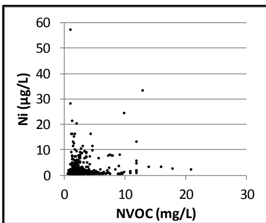
Bilag 17. Lokalenhed Fyn. Nikkel (Ni) vs dybde, nikkel og pH, nikkel og ilt (O 2 ), nikkel og nitrat (NO 3 ) samt nikkel og NVOC. Data er indsamlet i perioden 1993-2013 fra aktive borer i 2013. Koncentrationer under detektionsgrænsen er vist med den numeriske værdi.
