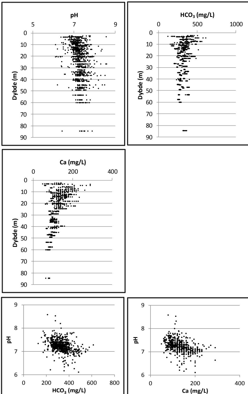
Bilag 1. Lokalenhed Fyn. pH, hydrogencarbonat (HCO 3 ) og calcium (Ca) vs dybde, pH og hydrogencarbonat samt pH og calcium. Data er indsamlet i perioden 1993-2013 fra aktive boringer i 2013. Koncentrationer under detektionsgrænsen er vist med den numeriske værdi.
