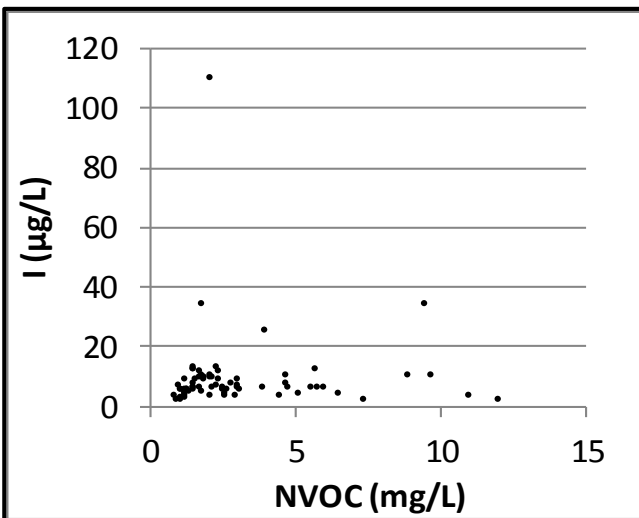
Bilag 16. Lokalenhed Fyn. Jod (I) vs dybde, jod og NVOC samt jod og chlorid (Cl). Data er indsamlet i perioden 1993-2013 fra aktive boringer i 2013. Koncentrationer under detektionsgrænsen er vist med den numeriske værdi.
