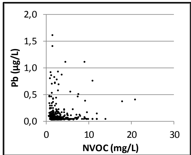
Bilag 18. Lokalenhed Fyn. Bly (Pb) vs dybde, bly og pH samt bly og NVOC. Data er indsamlet i perioden 1993-2013 fra aktive boringer i 2013. Koncentrationer under detektionsgrænsen er vist med den numeriske værdi.
