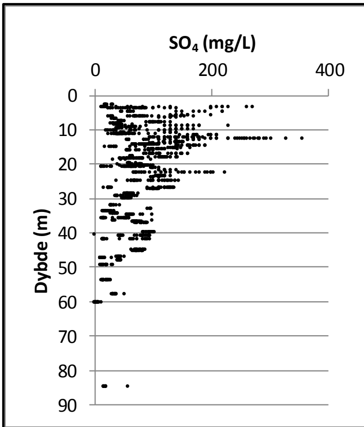
Bilag 6. Lokalenhed Fyn. Sulfat ( \text{SO}_4 ) vs. dybde. Data er indsamlet i perioden 1993-2013 fra aktive boringer i 2013. Koncentrationer under detektionsgrænsen er vist med den numeriske værdi.
