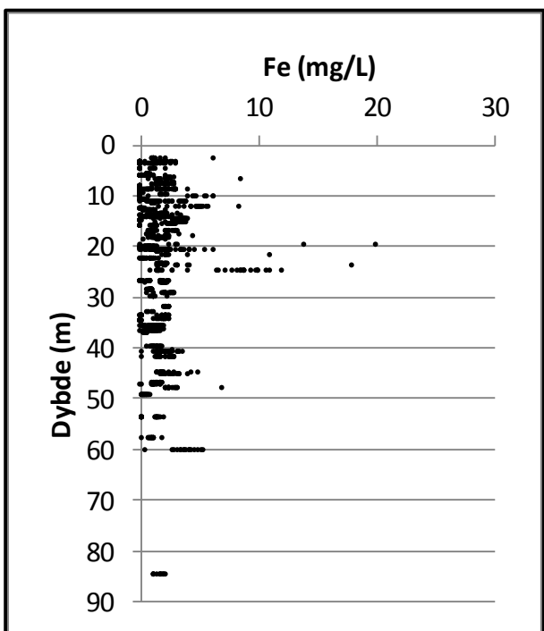
Bilag 2. Lokalenhed Fyn. Redoxpotentiale, ilt og jern vs dybde. Data er indsamlet i perioden 1993-2013 fra aktive borer i 2013. Koncentrationer under detektionsgrænsen er vist med den numeriske værdi.
