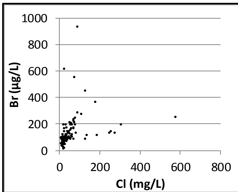
Bilag 12. Lokalenhed 3 Fyn. Brom (Br) vs dybde samt brom og chlorid (Cl). Data er indsamlet i perioden 1993-2013 fra aktive borer i 2013. Koncentrationer under detektionsgrænsen er vist med den numeriske værdi.
