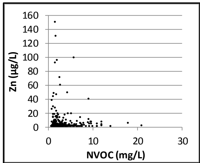
Bilag 19. Lokalenhed Fyn. Zink (Zn) vs dybde, zink og pH samt zink og NVOC. Data er indsamlet i perioden 1993-2013 fra aktive boringer i 2013. Koncentrationer under detektionsgrænsen er vist med den numeriske værdi.
