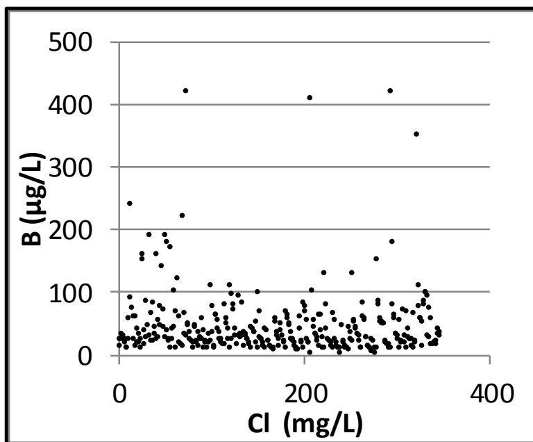
Bilag 9. Lokalenhed 3 Fyn. Bor (B) vs dybde samt bor og chlorid (Cl). Data er indsamlet i perioden 1993-2013 fra aktive boringer i 2013. Koncentrationer under detektionsgrænsen er vist med den numeriske værdi.
