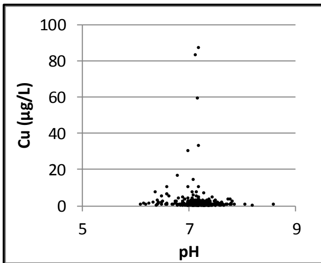
Bilag 14. Lokalenhed Fyn. Kobber (Cu) vs dybde, kobber og pH samt kobber og NVOC. Data er indsamlet i perioden 1993-2013 fra aktive borer i 2013. Koncentrationer under detektionsgrænsen er vist med den numeriske værdi.
