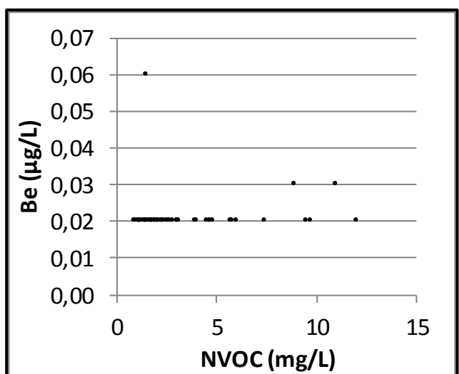
Bilag 11. Lokalenhed 3 Fyn. Beryllium (Be) vs dybde, beryllium og pH samt beryllium og NVOC. Data er indsamlet i perioden 1993-2013 fra aktive boringer i 2013. Koncentrationer under detektionsgrænsen er vist med den numeriske værdi.
