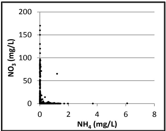
Bilag 2 Lokalenhed Fyn. Ilt ( O_2 ) og jern (Fe), ilt og ammonium ( NH_4 ), nitrat ( NO_3 ) og jern samt nitrat og ammonium. Data er indsamlet i perioden 1993-2013 fra aktive boringer i 2013. Koncentrationer under detektionsgrænsen er vist med den numeriske værdi.
