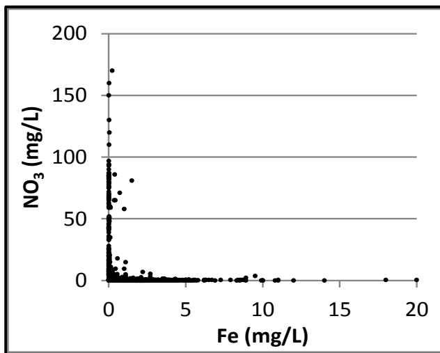
Bilag 2 Lokalenhed Fyn. Ilt ( O_2 ) og jern (Fe), ilt og ammonium ( NH_4 ), nitrat ( NO_3 ) og jern samt nitrat og ammonium. Data er indsamlet i perioden 1993-2013 fra aktive boringer i 2013. Koncentrationer under detektionsgrænsen er vist med den numeriske værdi.
