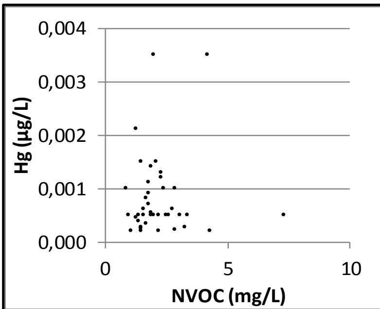
Bilag 15. Lokalenhed Fyn. Kviksølv (Hg) vs dybde og kviksølv og NVOC. Data er indsamlet i perioden 1993-2013 fra aktive boringer i 2013. Koncentrationer under detektionsgrænsen er vist med den numeriske værdi.
