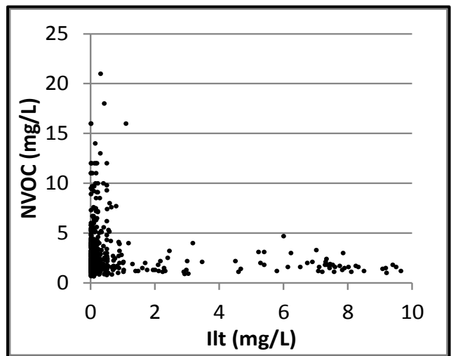
Bilag 4. Lokalenhed Fyn. NVOC vs. dybde, NVOC og ilt ( O_2 ) samt NVOC og pH. Data er indsamlet i perioden 1993-2013 fra aktive boringer i 2013. Koncentrationer under detektionsgrænsen er vist med den numeriske værdi.
