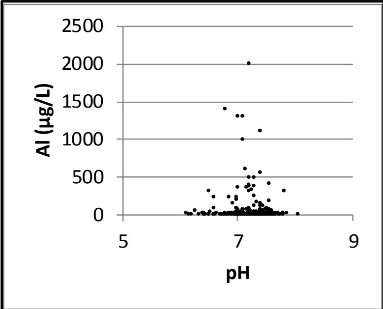
Bilag 7. Lokalenhed Fyn. Aluminium (Al) vs dybde samt aluminium og pH. Data er indsamlet i perioden 1993-2013 fra aktive boringer i 2013. Koncentrationer under detektionsgrænsen er vist med den numeriske værdi.
