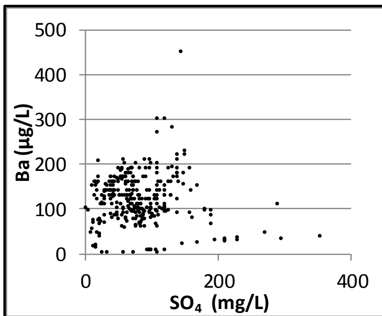
Bilag 10. Lokalenhed 3 Fyn. Barium vs dybde samt barium og sulfat ( \text{SO}_4 ). Data er indsamlet i perioden 1993-2013 fra aktive borer i 2013. Koncentrationer under detektionsgrænsen er vist med den numeriske værdi.
