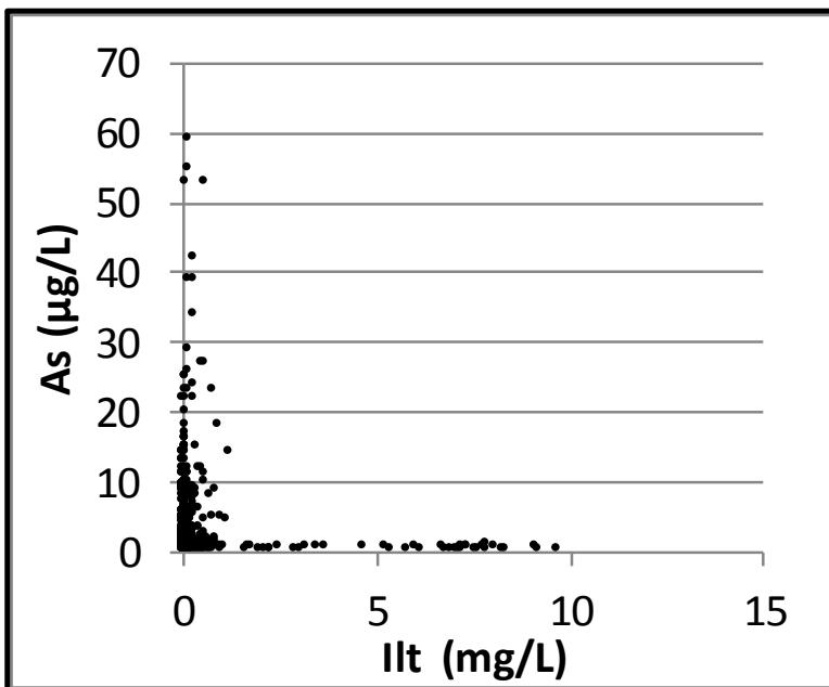
Bilag 8. Lokalenhed Fyn. Arsen vs dybde samt arsen og ilt ( \text{O}_2 ). Data er indsamlet i perioden 1993-2013 fra aktive borer i 2013. Koncentrationer under detektionsgrænsen er vist med den numeriske værdi.
