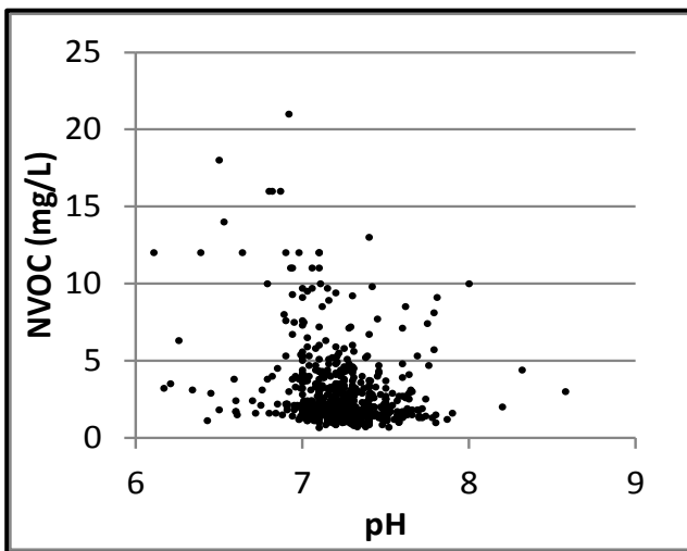
Bilag 4. Lokalenhed Fyn. NVOC vs. dybde, NVOC og ilt ( O_2 ) samt NVOC og pH. Data er indsamlet i perioden 1993-2013 fra aktive boringer i 2013. Koncentrationer under detektionsgrænsen er vist med den numeriske værdi.
