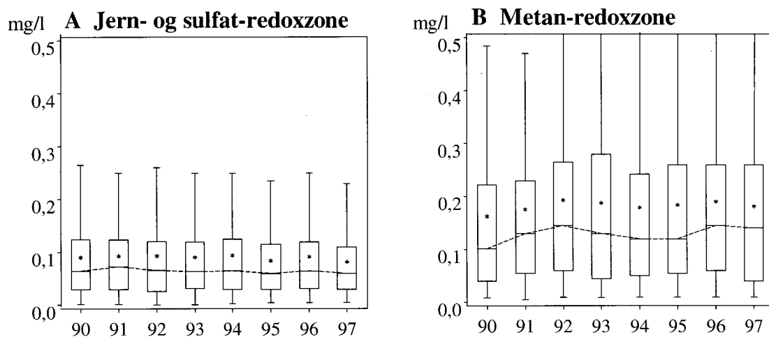
Figur 2.8 Box-plot med fosforudviklingen i jern- og sulfat-redoxzonen og i metan-redoxzonen i perioden 1990 – 1997 baseret på data fra alle aktive filtre i GRUMO.
