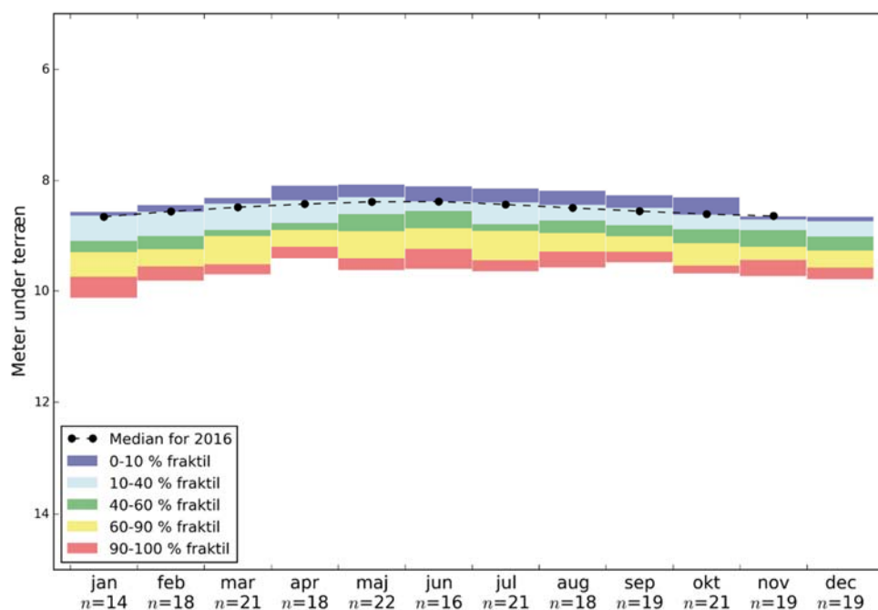
Figur 1.2 Pejletidsserier (vandstand m u. t.) månedsmedian for 2016 s i forhold til med månedsværdier 1990-2015, DGU nr. 76.853, Midtjylland. n= antal år med målinger i en måned.
