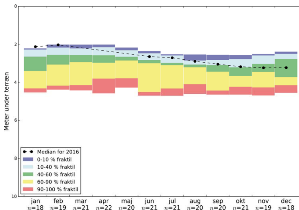
Figur 1.3. Pejletidsserier (vandstand m u. t.) månedsmedian for 2016 i forhold til t med månedsværdier 1990-2015, DGU nr. 166.485, Sønderjylland. n= antal år med målinger i en måned.
