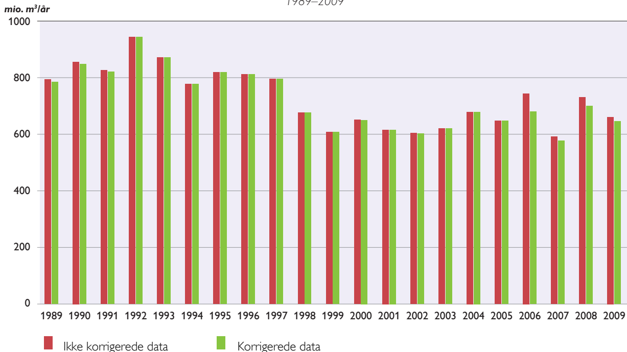
Figur 38. De røde søjler viser den samlede grundvandsindvinding i Danmark (mio. m 3 /år) alene baseret på indberetninger til GEUS uden nogen form for korrektion. De grønne søjler viser data korrigerede for fejlindberetninger.
