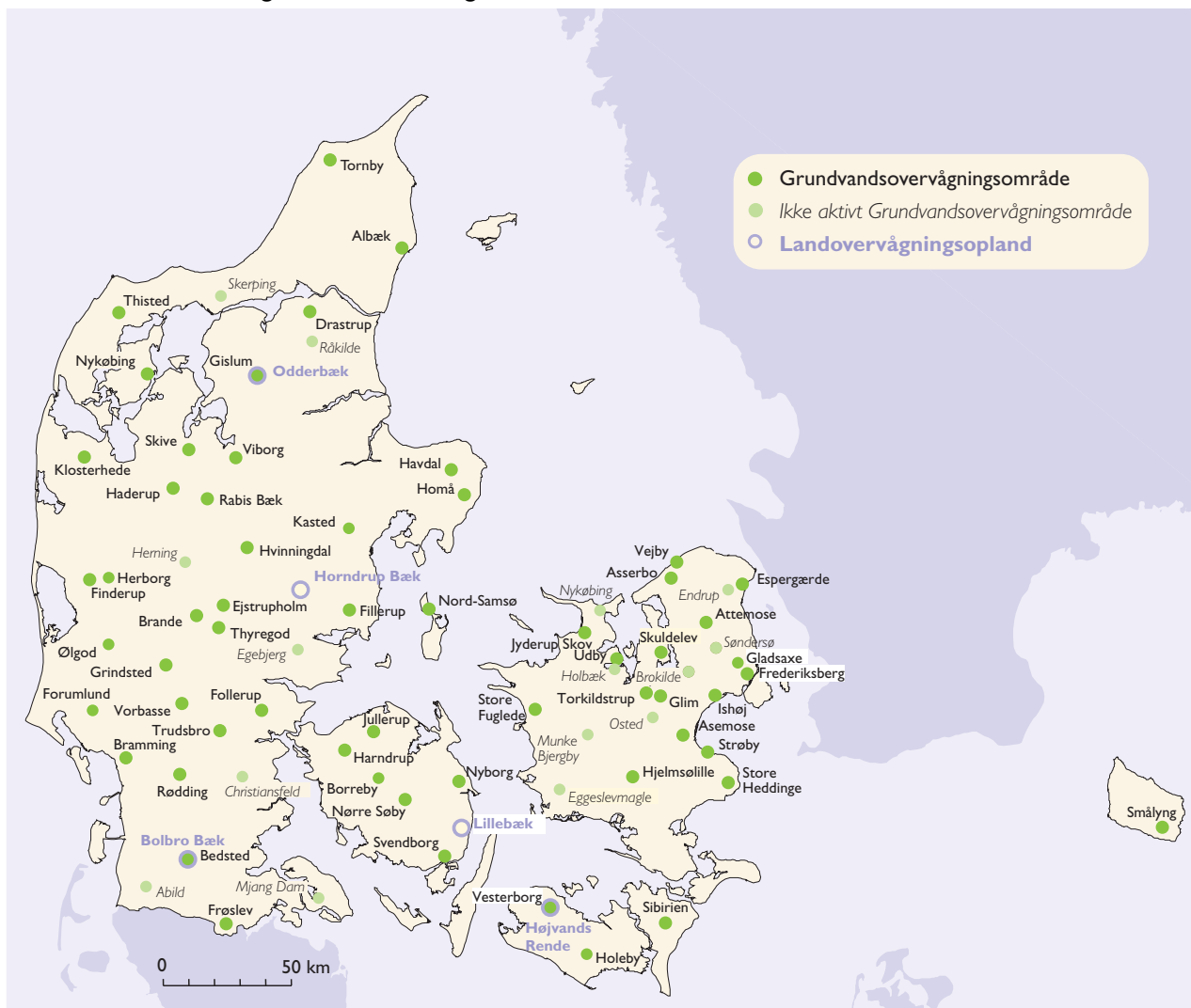
Figur 1. Grundvandsovervågningen i Danmark i 2007-2009 omfatter vandanalyser fra 62 grundvandsovervågnings-områder (GRUMO) og 5 landovervågningsoplande (LOOP). I 6 områder er der etableret en redoxboring til overvågning af de kemiske forhold omkring redoxzonerne. Landovervågnings-oplandene består af tre ler-oplande (Horndrup Bæk, Lillebæk og Højvads Rende) og to sand-oplande (Oddebæk og Bolbro Bæk).
