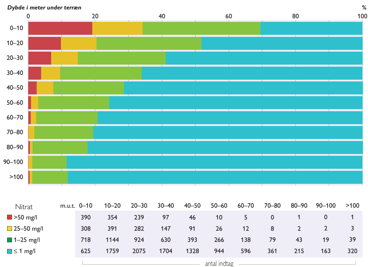
Dybdemæssig fordeling af det gennemsnitlige nitratindehold Alle analyser 1990–2009
