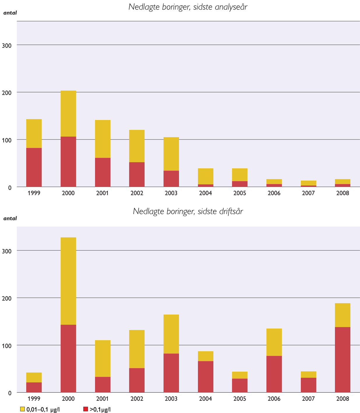
Figur 29. Indvindingsboringer, med pesticidindhold, taget ud af drift i perioden 1999 til 2008. Figur 29 nederst viser sidste driftsår – altså sidste gang, boringen forekom i et boringskontroldatasæt (dvs. lukningen ikke nødvendigvis skyldes en pesticidanalyse). Stigningen i 2008 skyldes formodentlig indberetningen af ældre analyser, og derfor stammer nogle af boringerne fra 2008 sandsynligvis fra de foregående år . Figur 29 øverst viser sidste gang, en boring optræder med en pesticidanalyse i et boringskontroldatasæt. Boringerne kan være taget ud af drift af andre årsager end forekomst af pesticider eller nedbrydningsprodukter fra disse, fx overskridelse af kvalitetskrav for nitrat eller af tekniske årsager mm. Fra Brüsich (2010).
