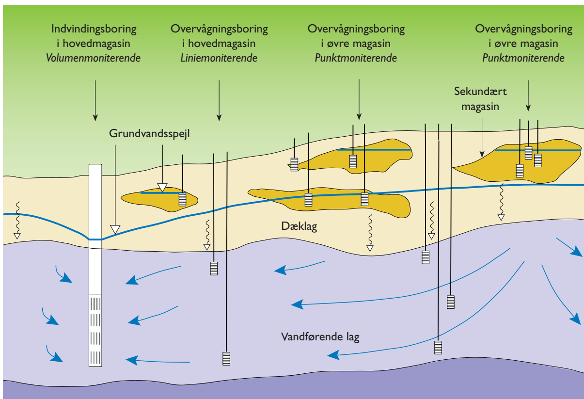
Figur 2. Principskitse for et grundvandsovervågningsområde (efter Andersen 1987).
