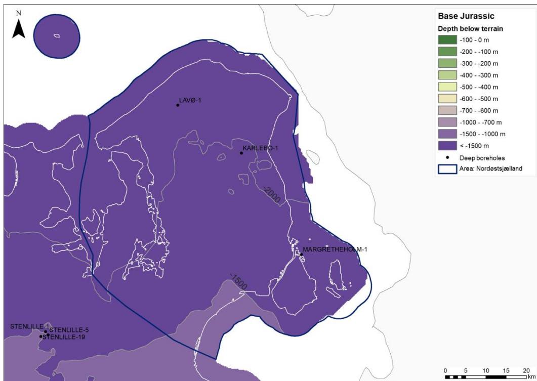
Figure 6.136. Base Jurassic depth map, Nordøstsjælland area.
