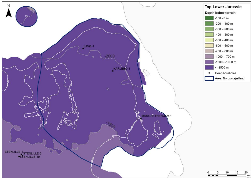
Figure 6.135. Top Lower Jurassic depth map, Nordøstsjælland area.
