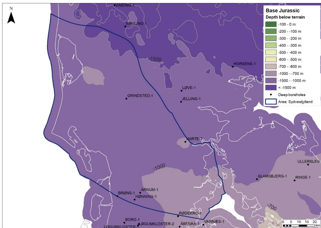
Figure 6.65. Base Jurassic depth map, Sydvestjylland area.
