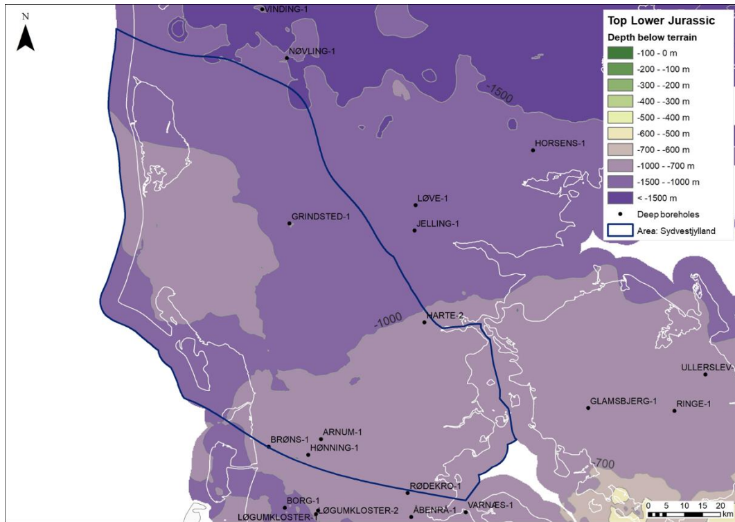
Figure 6.64. Top Lower Jurassic depth map, Sydvestjylland area.
