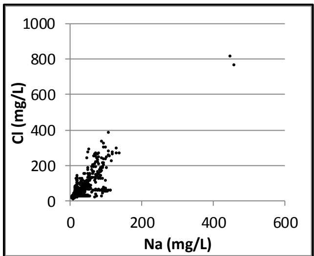
Bilag 3. Lokalenhed Nordjylland. Chlorid (Cl) vs. dybde, chlorid og ledningsevne samt chlorid og natrium (Na). Data er indsamlet i perioden 1993-2013 fra aktive borer i 2013. Koncentrationer under detektionsgrænsen er vist med den numeriske værdi.
