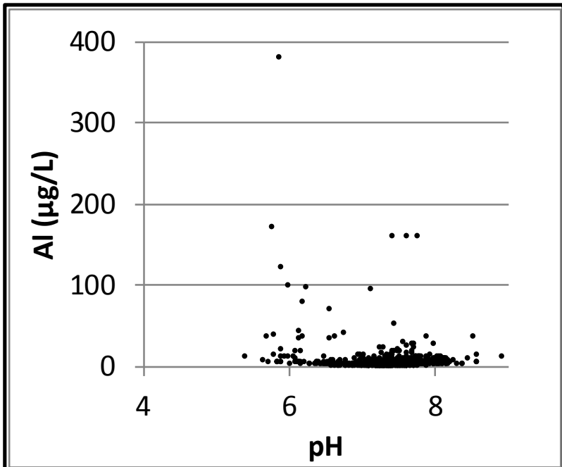
Bilag 7. Lokalenhed Nordjylland. Aluminium (Al) vs dybde samt aluminium og pH. Data er indsamlet i perioden 1993-2013 fra aktive borer i 2013. Koncentrationer under detektionsgrænsen er vist med den numeriske værdi.
