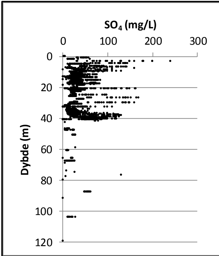
Bilag 6. Lokalenhed Nordjylland. Sulfat ( \text{SO}_4 ) vs. dybde. Data er indsamlet i perioden 1993-2013 fra aktive boringer i 2013. Koncentrationer under detektionsgrænsen er vist med den numeriske værdi.
