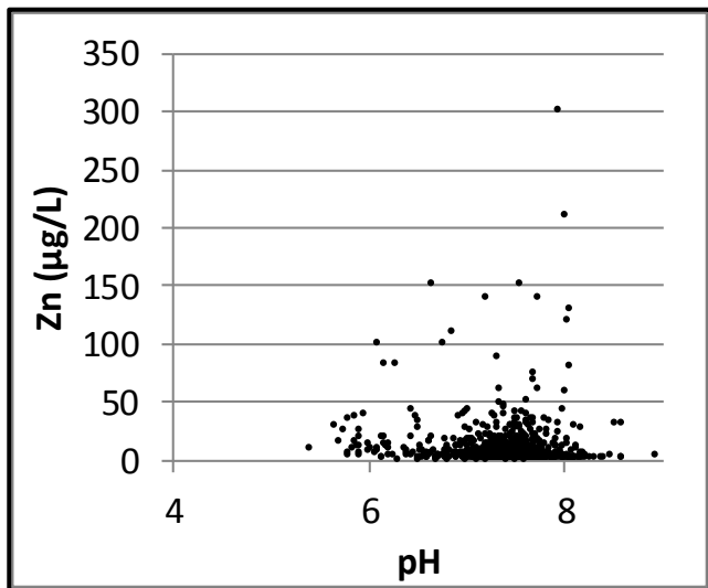
Bilag 19. Lokalenhed Nordjylland. Zink (Zn) vs dybde, zink og pH samt zink og NVOC. Data er indsamlet i perioden 1993-2013 fra aktive borer i 2013. Koncentrationer under detektionsgrænsen er vist med den numeriske værdi.
