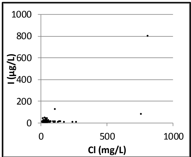
Bilag 16. Lokalenhed Nordjylland. Jod (I) vs dybde, jod og NVOC samt jod og chlorid (Cl). Data er indsamlet i perioden 1993-2013 fra aktive boringer i 2013. Koncentrationer under detektionsgrænsen er vist med den numeriske værdi.
