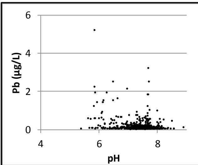
Bilag 18. Lokalenhed Nordjylland. Bly (Pb) vs dybde, bly og pH samt bly og NVOC. Data er indsamlet i perioden 1993-2013 fra aktive boringer i 2013. Koncentrationer under detektionsgrænsen er vist med den numeriske værdi.
