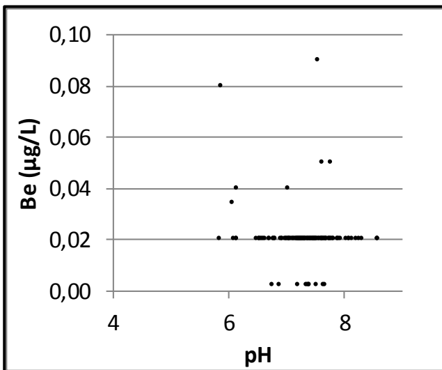
Bilag 11. Lokalenhed Nordjylland. Beryllium (Be) vs dybde, beryllium og pH samt beryllium og NVOC. Data er indsamlet i perioden 1993-2013 fra aktive boringer i 2013. Koncentrationer under detektionsgrænsen er vist med den numeriske værdi.
