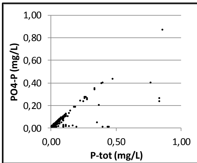
Bilag 5. Lokalenhed Nordjylland. Phosphat ( \text{PO}_4\text{-P} ) og total-fosfor ( \text{P-tot} ) vs. dybde samt \text{PO}_4\text{-P} og \text{P-tot} . Data er indsamlet i perioden 1993-2013 fra aktive boringer i 2013. Koncentrationer under detektionsgrænsen er vist med den numeriske værdi.
