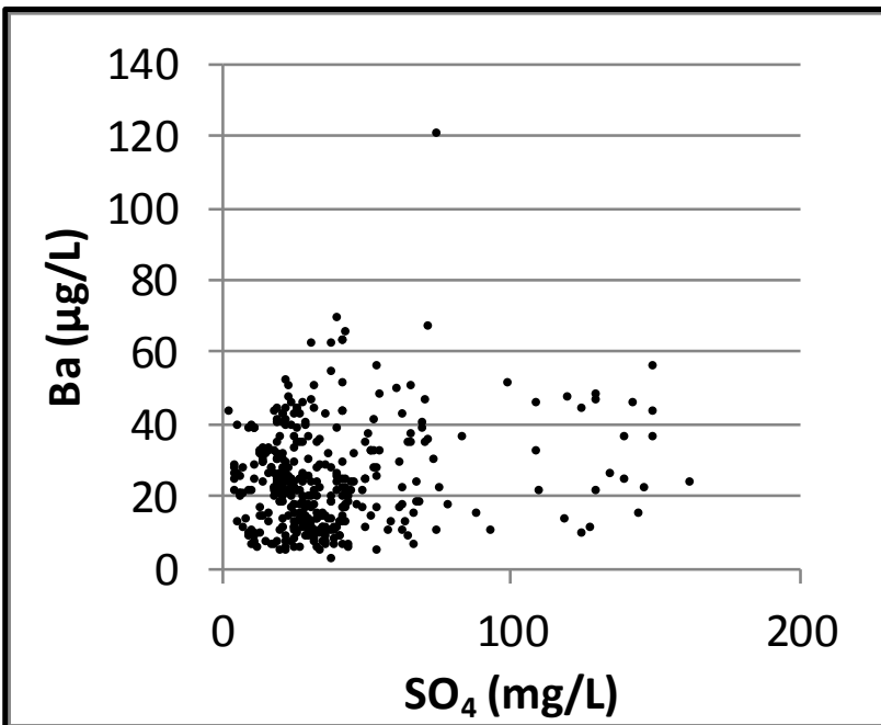
Bilag 10. Lokalenhed Nordjylland. Barium vs dybde samt barium og sulfat (SO 4 ). Data er indsamlet i perioden 1993-2013 fra aktive borer i 2013. Koncentrationer under detektionsgrænsen er vist med den numeriske værdi.
