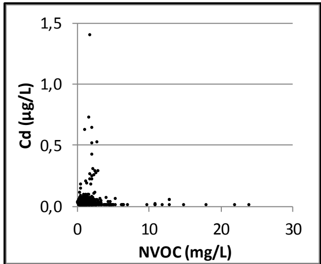
Bilag 13. Lokalenhed Nordjylland. Cadmium (Cd) vs dybde, cadmium og pH samt cadmium og NVOC. Data er indsamlet i perioden 1993-2013 fra aktive boringer i 2013. Koncentrationer under detektionsgrænsen er vist med den numeriske værdi.
