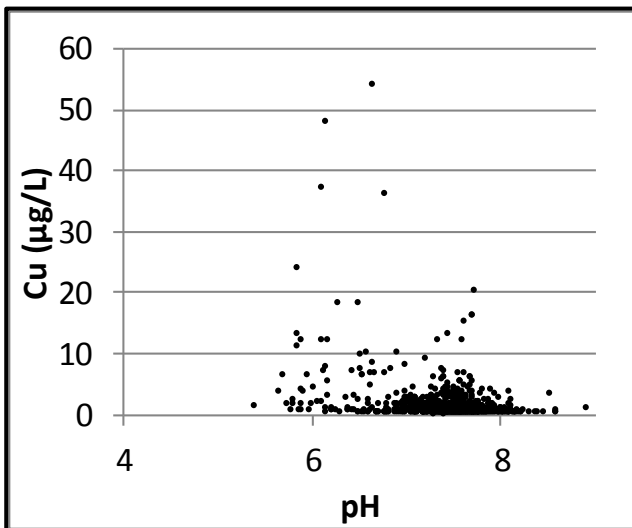
Bilag 14. Lokalenhed Nordjylland. Kobber (Cu) vs dybde, kobber og pH samt kobber og NVOC. Data er indsamlet i perioden 1993-2013 fra aktive boringer i 2013. Koncentrationer under detektionsgrænsen er vist med den numeriske værdi.
