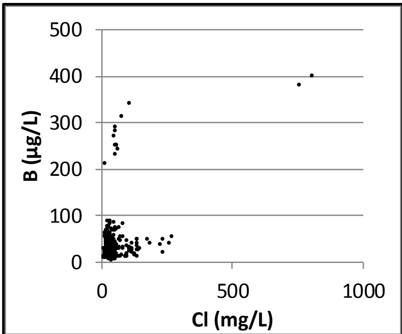
Bilag 9. Lokalenhed Nordjylland. Bor (B) vs dybde samt bor og chlorid (Cl). Data er indsamlet i perioden 1993-2013 fra aktive boringer i 2013. Koncentrationer under detektionsgrænsen er vist med den numeriske værdi.
