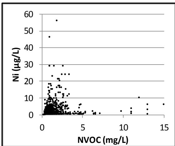
Bilag 17. Lokalenhed Nordjylland. Nikkel (Ni) vs dybde, nikkel og pH, nikkel og ilt (O 2 ), nikkel og nitrat (NO 3 ) samt nikkel og NVOC. Data er indsamlet i perioden 1993-2013 fra aktive borer i 2013. Koncentrationer under detektionsgrænsen er vist med den numeriske værdi.
