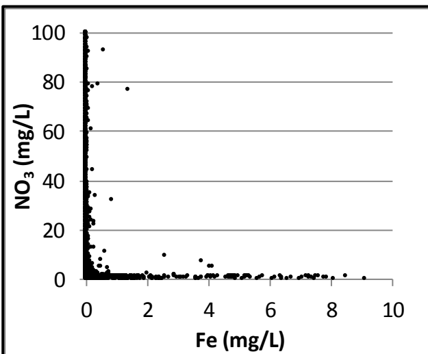
Bilag 2. Lokalenhed Nordjylland. Ilt ( O_2 ) og jern (Fe), ilt og ammonium ( NH_4 ), nitrat ( NO_3 ) og jern samt nitrat og ammonium. Data er indsamlet i perioden 1993-2013 fra aktive borer i 2013. Koncentrationer under detektionsgrænsen er vist med den numeriske værdi.
