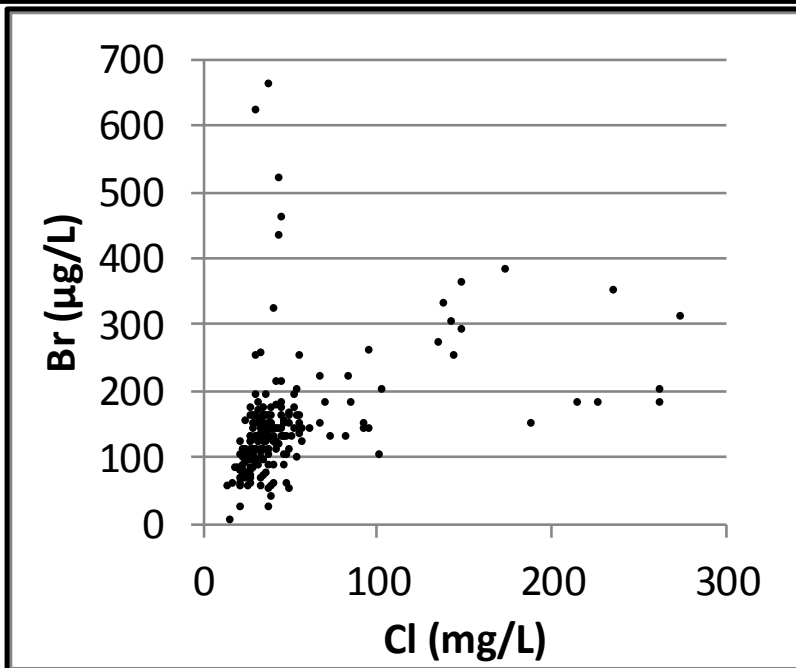
Bilag 12. Lokalenhed Nordjylland. Brom (Br) vs dybde samt brom og chlorid (Cl). Data er indsamlet i perioden 1993-2013 fra aktive borer i 2013. Koncentrationer under detektionsgrænsen er vist med den numeriske værdi.
