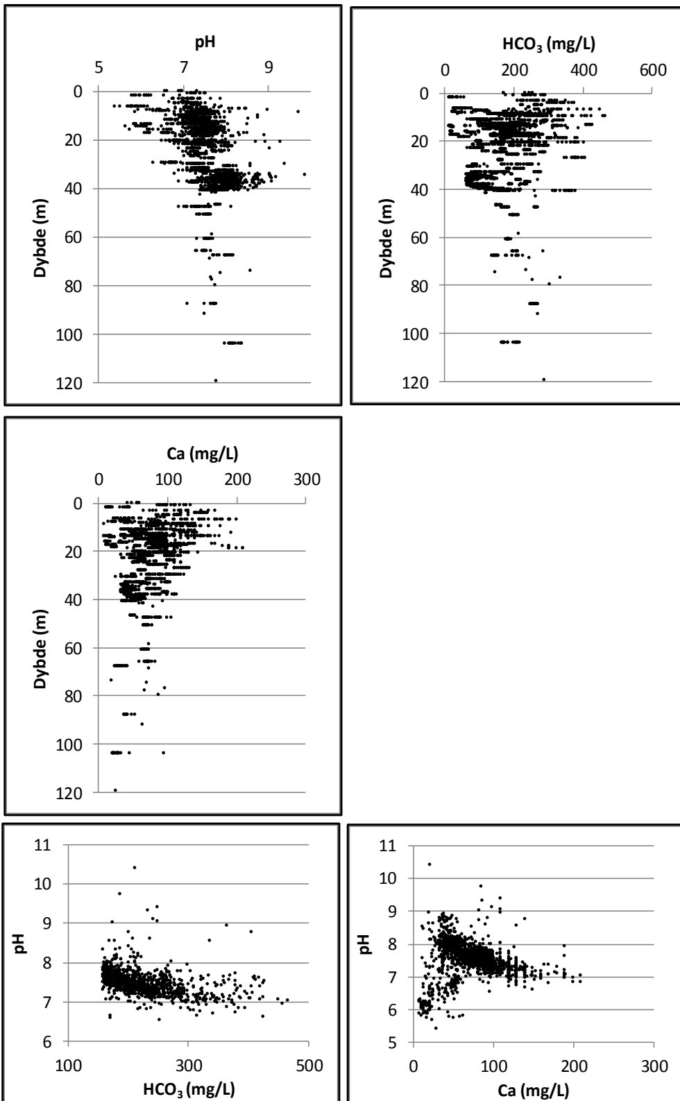
Bilag 1. Lokalenhed Nordjylland. pH, hydrogencarbonat (HCO 3 ) og calcium (Ca) vs dybde, pH og hydrogencarbonat samt pH og calcium. Data er indsamlet i perioden 1993-2013 fra aktive boringer i 2013. Koncentrationer under detektionsgrænsen er vist med den numeriske værdi.
