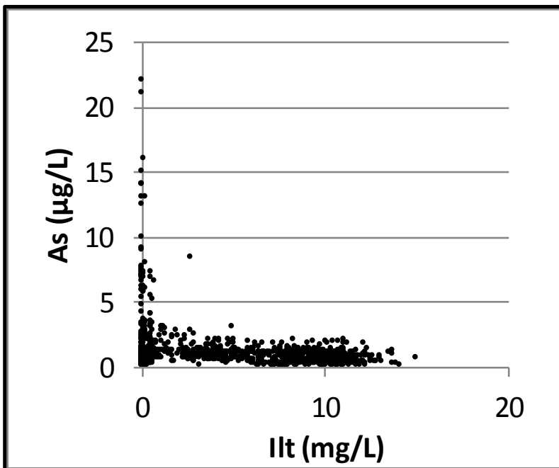
Bilag 8. Lokalenhed Nordjylland. Arsen vs dybde samt arsen og ilt ( \text{O}_2 ). Data er indsamlet i perioden 1993-2013 fra aktive boringer i 2013. Koncentrationer under detektionsgrænsen er vist med den numeriske værdi.
