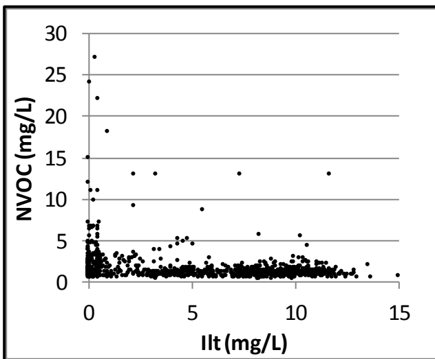
Bilag 4. Lokalenhed Nordjylland. NVOC vs. dybde, NVOC og ilt ( O_2 ) samt NVOC og pH. Data er indsamlet i perioden 1993-2013 fra aktive borer i 2013. Koncentrationer under detektionsgrænsen er vist med den numeriske værdi.
