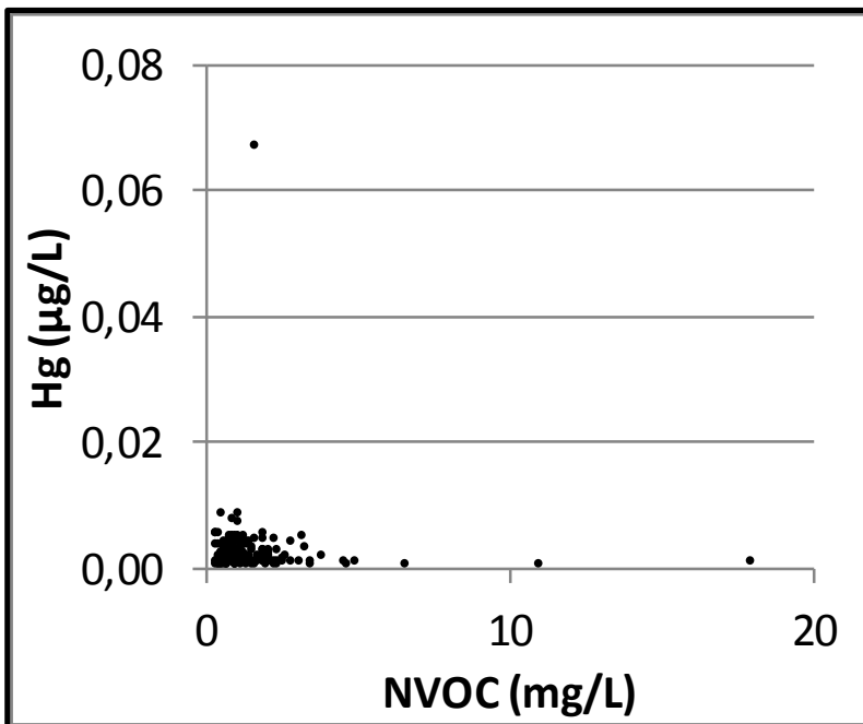
Bilag 15. Lokalenhed Nordjylland. Kviksølv (Hg) vs dybde og kviksølv og NVOC. Data er indsamlet i perioden 1993-2013 fra aktive boringer i 2013. Koncentrationer under detektionsgrænsen er vist med den numeriske værdi.
