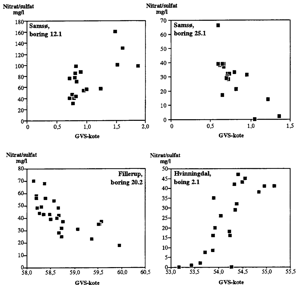
Figur 2.7 Nitratkoncentrationen i ustabile borer i Århus Amt (1999) som funktion af grundvandsspejlet.
