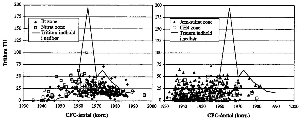
Figur 6.5. Tritiumindhold i grundvand vist som funktion af CFC-årstal. CFC-årstallene er korrigerede for forskel i analysetidspunkter. Hvis CFC-årstallet er bestemt til f.eks. 1950 og tritiumanalysen er udført otte år før CFC-analysen afsættes tritiumværdien ved 1942.
