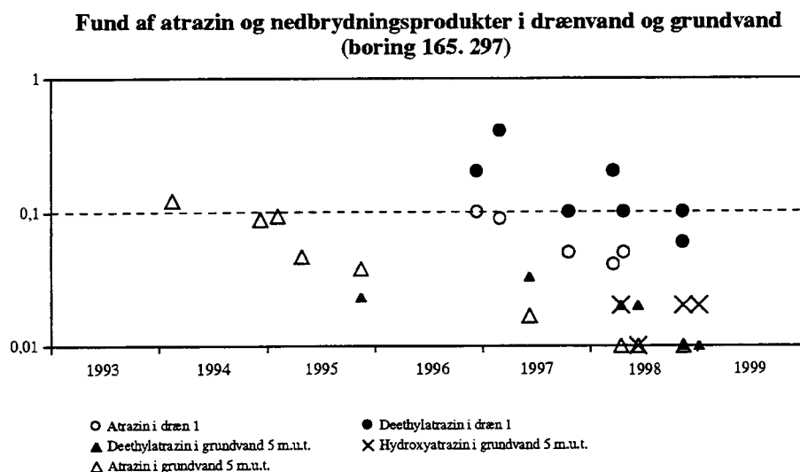
Figur 5.12 Koncentrationen (logaritmisk) af atrazin og nedbrydningsprodukter i drænvand og grundvand i LOOP 4 på Fyn i perioden 1994-1999.
