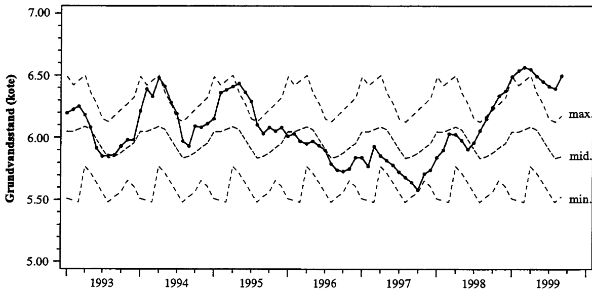
Figur 7.4 Grundvandsstand for 1993-99 for to pejlestationer på øerne fra det nationale pejlestationsnet (Vejstrup på Sydøstfyn og Villingerød i Nordsjælland) samt minimum, maksimum og middelværdier for perioden 1971-92 for de enkelte måneder (kilde: National Vandressource Model, http://www.vandmodel.dk ).
