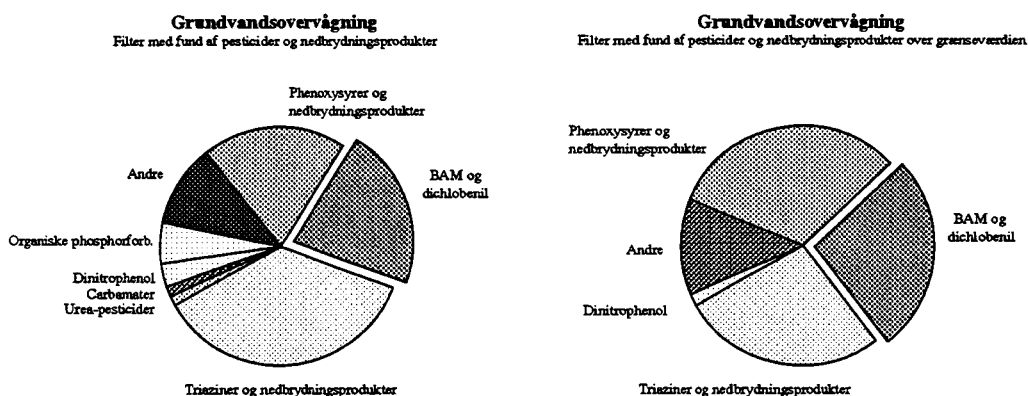
Figur 5.3 Filtre med fund af pesticider og nedbrydningsprodukter i grundvands-overvågningen i 1989-1998, beregnet på grundlag af bilag 5.1.
