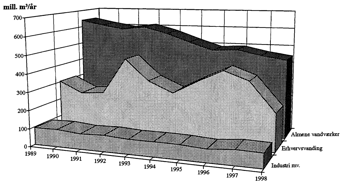
Figur 7.1 Vandindvinding i Danmark (mill. m 3 /år) fordelt på indvindingskategorier baseret på indberetninger til GEUS og oplysninger fra amternes overvågningsrapporter for perioden 1989-1998. Vandindvindingen i 1998, især til markvanding, var den laveste i mange år
