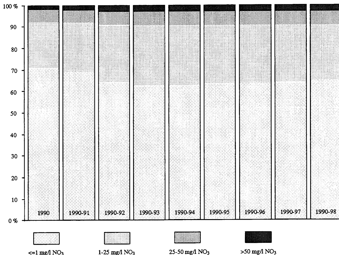
Figur 2.8 Summeret fordeling af nitratanalyser fra boringskontrollen. Perioden 1990-98 omfatter 5.669 boringer med under 1 mg/l nitrat, 2.162 boringer med nitratindhold mellem 1 og 25 mg/l nitrat, 553 boringer med nitrat mellem 25 og 50 mg/l nitrat og 246 boringer over 50 mg/l nitrat.
