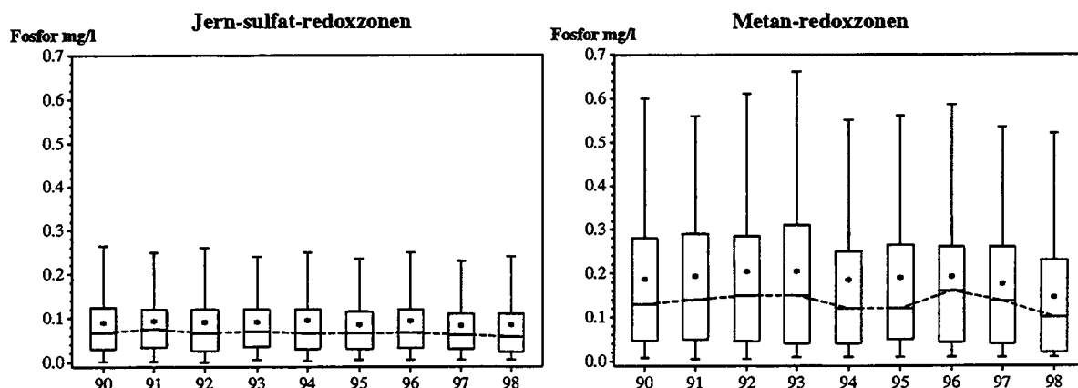
Figur 2.10 Box-plot med fosforudviklingen i jern- og sulfat-redoxzonen og i metan-redoxzonen i perioden 1990 – 1998 baseret på data fra alle aktive filtre i GRUMO.
