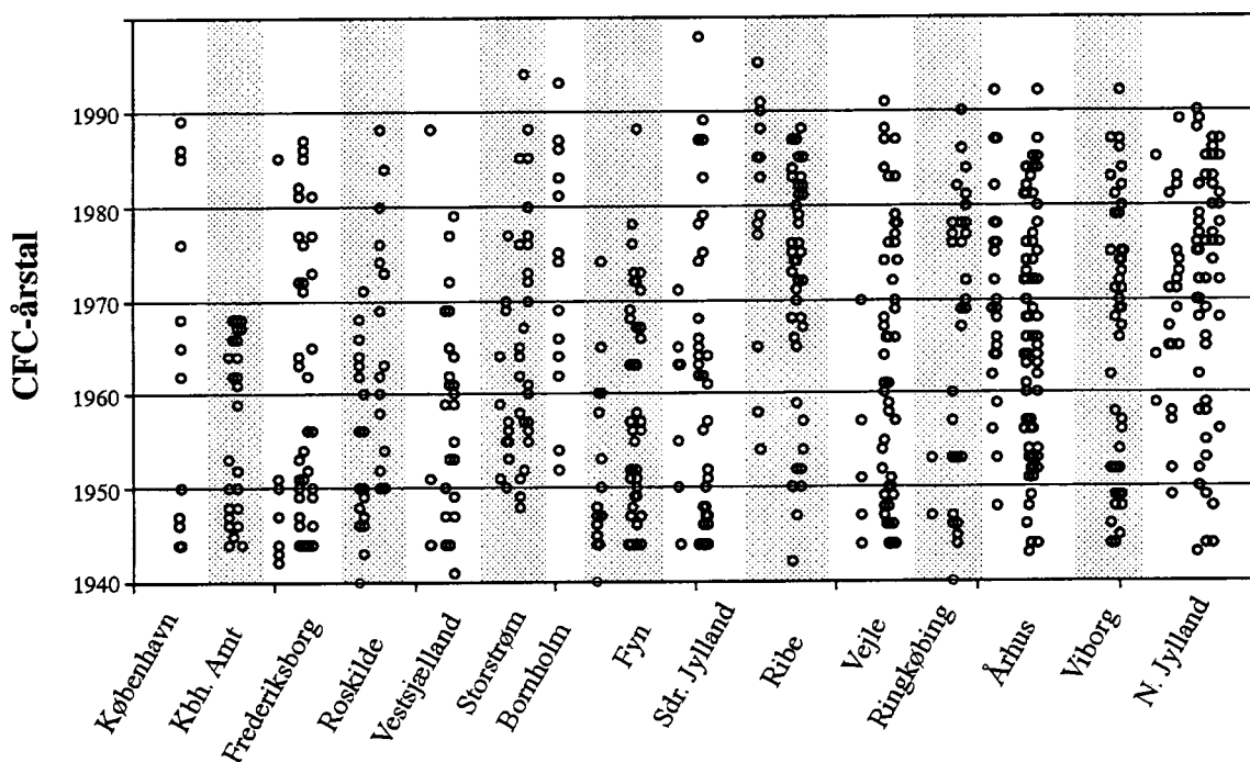
Figur 6.3 Resultaterne af CFC-dateringerne af grundvand i overvågningsområderne.
