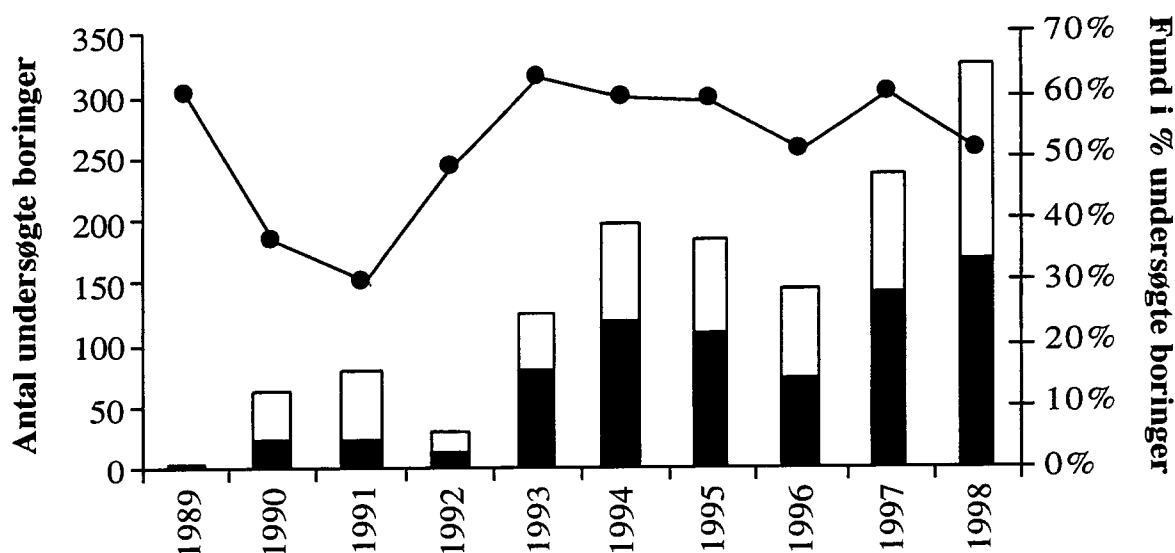
Figur 4.5 Fund af anioniske detergenter i vandværkernes boringskontrol i perioden 1989-1998. Total antal undersøgte boringer er vist som sum af undersøgte boringer uden fund (□) og med fund (■). Kurven (●) angiver hyppighed af fund som procent af antal boringer.
