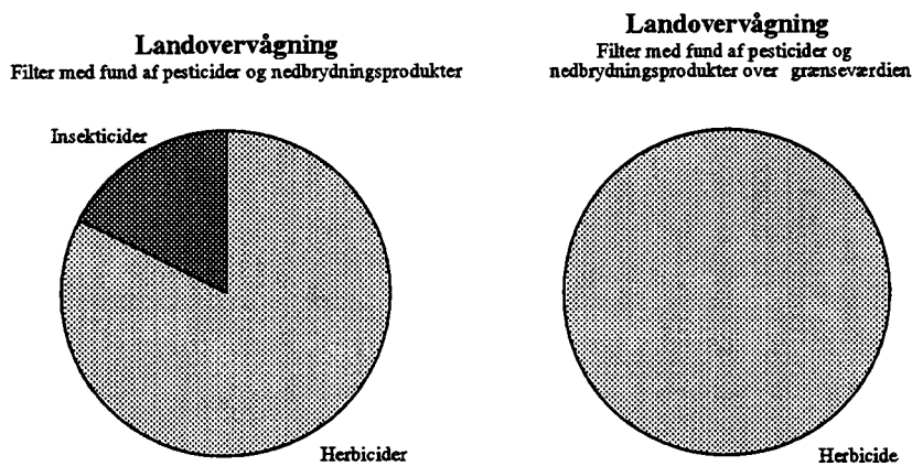
Figur 5.11 Filtre med fund af pesticider og nedbrydningsprodukter i landovervågningen i 1990-1999.
