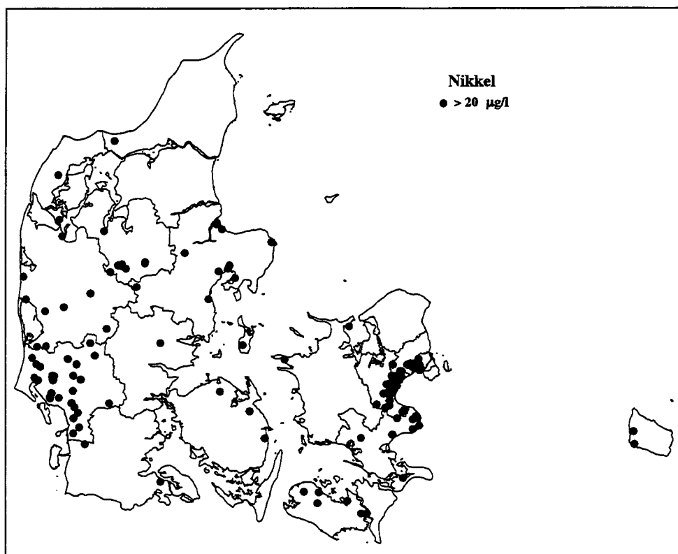
Figur 3.1 Vandforsyningsboringer med nikkelinhold over 20 µg/l. Grænseværdien for nikkel i drikkevand er 20 µg/l ved fraløb fra vandværk
